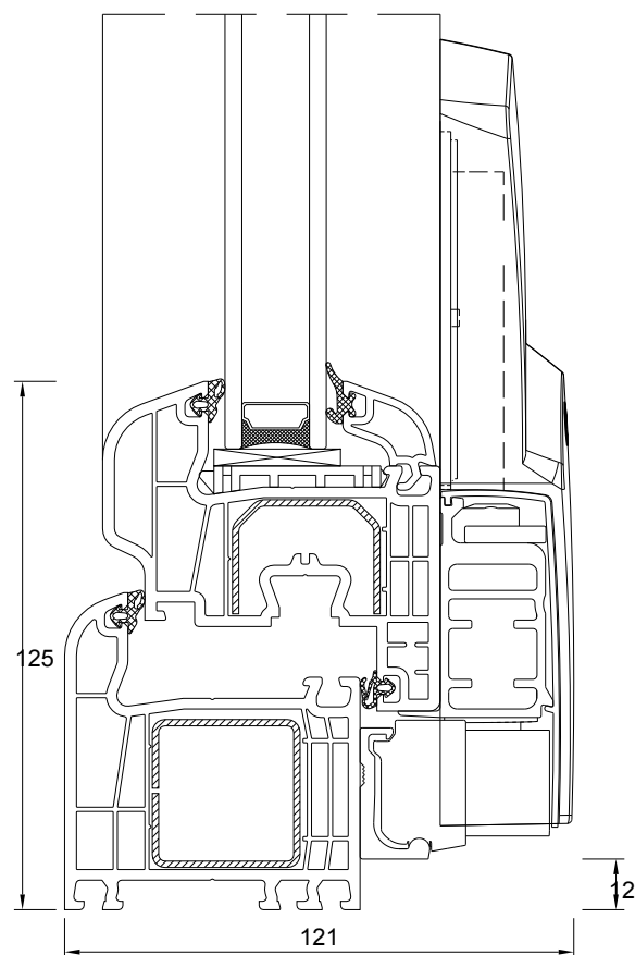
B - B
